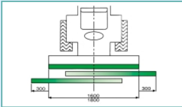
Con spostamento idraulico o manuale. With hydraulic or manual side offset. Avec deport manuel ou hydraulique. Mit mechanischer, oder hydraulischer Seitenverschiebung
